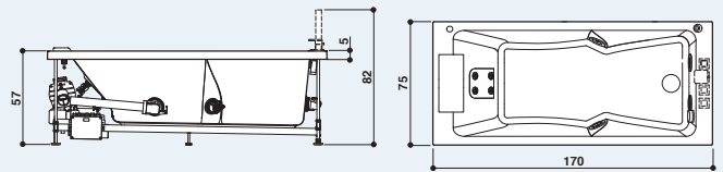
Left hand version view · Vue de la version gauche Abb. Linksausführung · Вид модели в левостороннем исполнении
